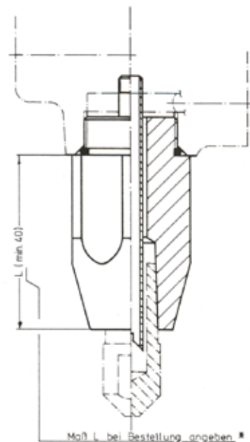
Prodloužení držáku elektrody
