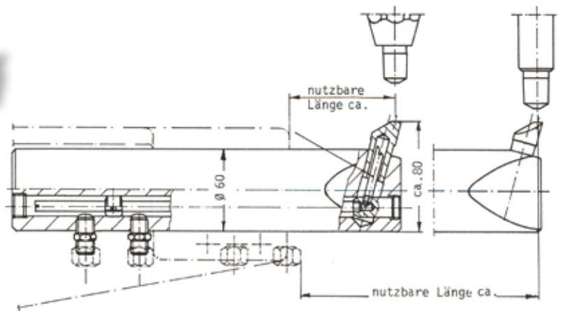
Trubková ramena pro konkrétní typy strojů Ø 60 / šikmá elektroda
