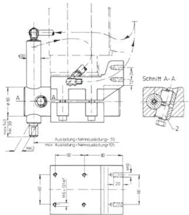
Předsunutý držák elektrody
