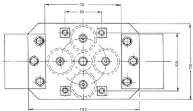
Vyrovnávací plato přitlaku pro přípr. výstup. svařovacích lisů / max. síla: 1200 daN
