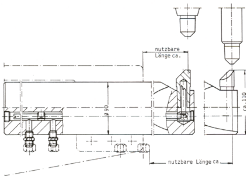
Trubková ramena pro konkrétní typy strojů Ø 90 / přímá elektroda
