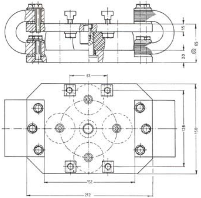
Vyrovnávací plato přítlaču pro přípr. výstup. svařovacích lisů / max. síla: 1800 daN
