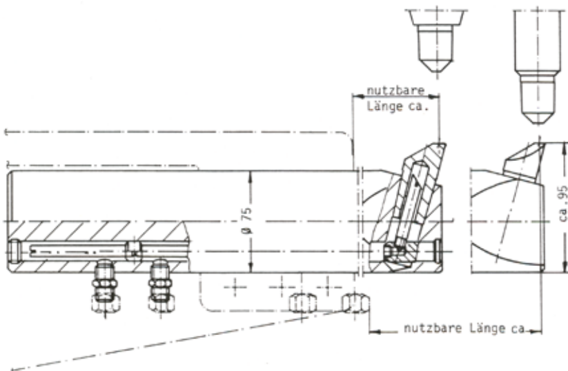
Trubková ramena pro konkrétní typy strojů Ø 75 / šikmá elektroda
