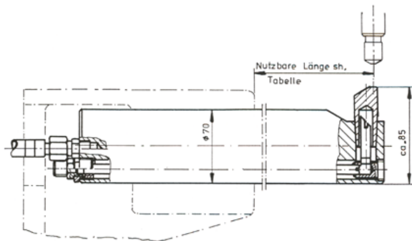
Trubková ramena pro konkrétní typy strojů Ø 70 / přímá elektroda
