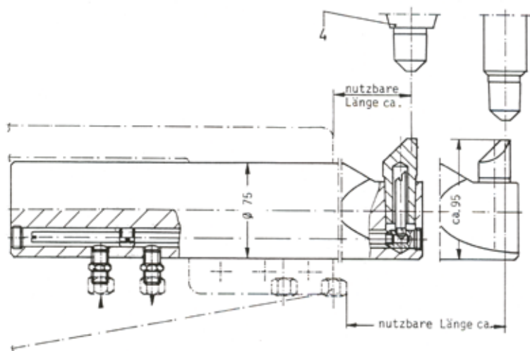
Trubková ramena pro konkrétní typy strojů Ø 75 / přímá elektroda
