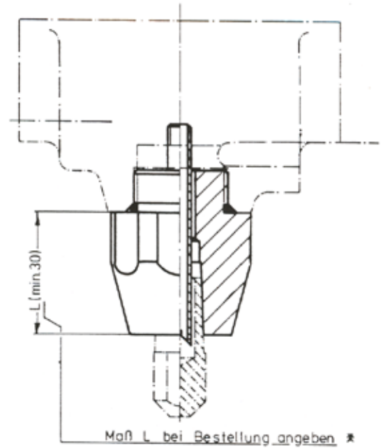
Prodloužení držáku elektrody
