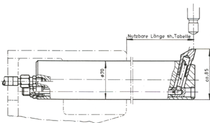
Trubková ramena pro konkrétní typy strojů Ø 70 / šikmá elektroda
