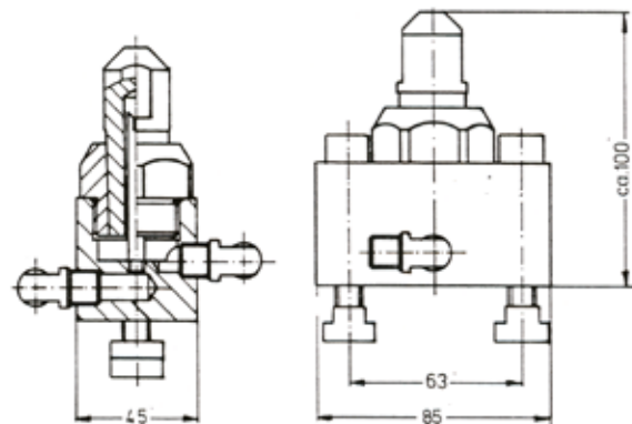
Přírubový držák elektrody
