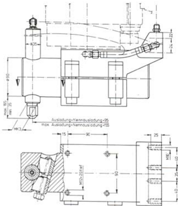
Předsunutý držák elektrody
