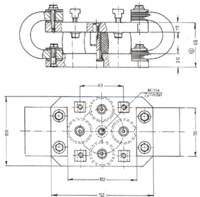
Vyrovnávací plato přítlaču pro přípr. výstup. svařovacích lisů / max. síla: 700 daN
