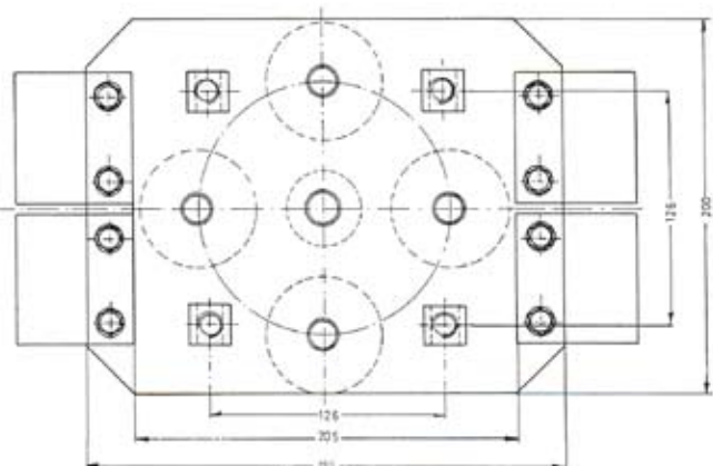
Vyrovnávací plato přitlaku pro přípr. výstup. svařovacích lisů / max. síla: 3000 daN
