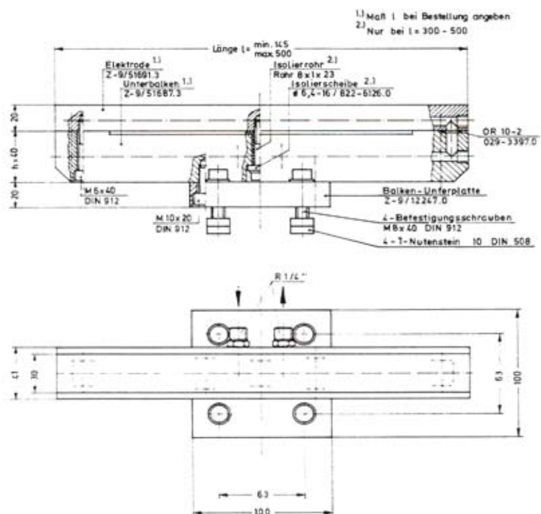
Samostatná plochá elektroda
