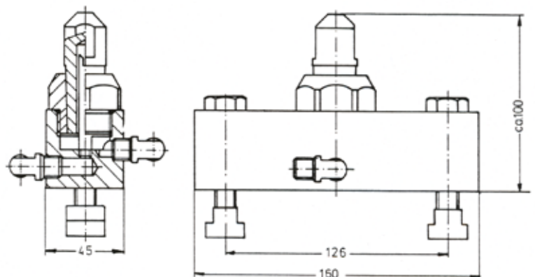
Přírubový držák elektrody připojení chlazení 1/4 / připojení chlaz. M16 x 1,5
