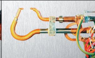
ROBOTOVÉ-C-KLEŠTĚ
